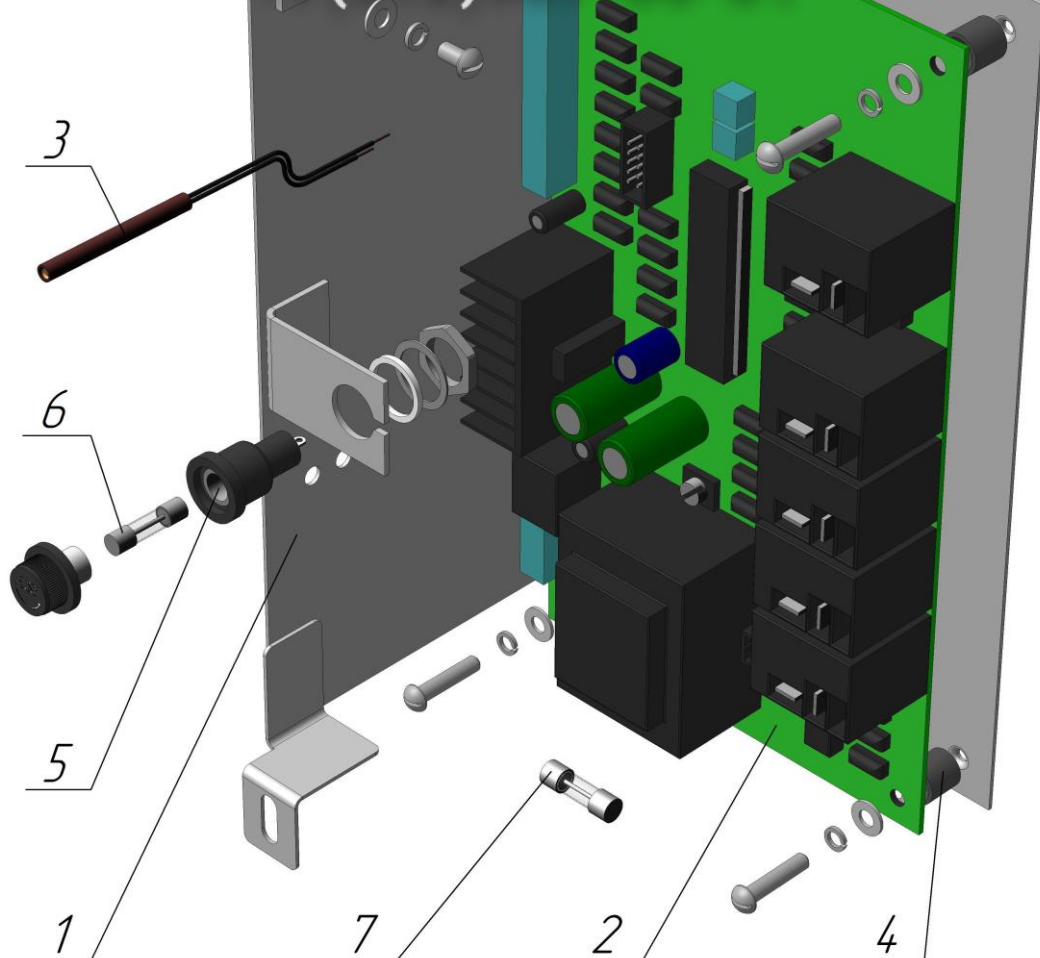
Рисунок 8. Панели МПФ 65.000 и МПФ 65.000-01
