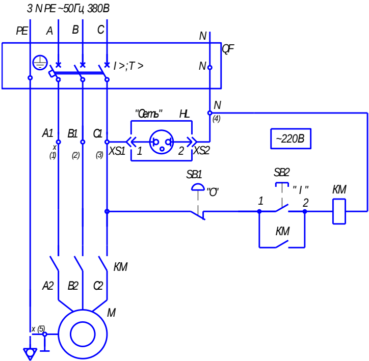
QF - Выключатель автоматический; KM - Пускатель магнитный; HL - Индикатор; М - Электродвигатель; SB1 - Кнопка «СТОП»; SB2 - Кнопка «ПУСК»; X - Блок зажимов; XS1, XS2 - Соединители
