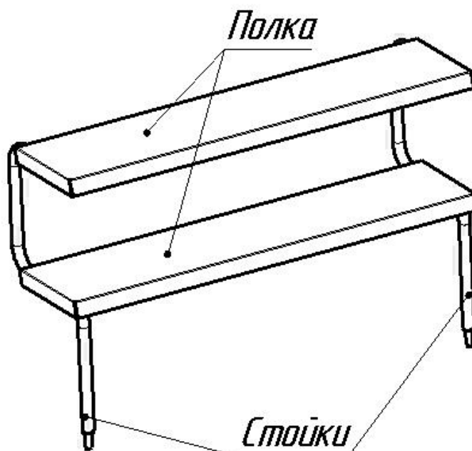
Рис.4 – Полка двойная
