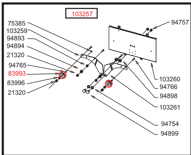
VECCHIA CONFIGURAZIONE
