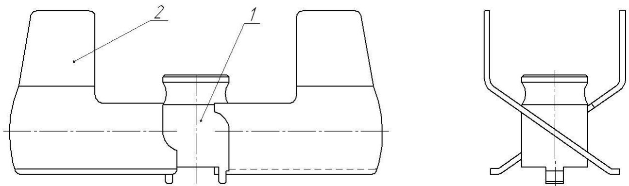
Рисунок 15 – Ротор лопастной
