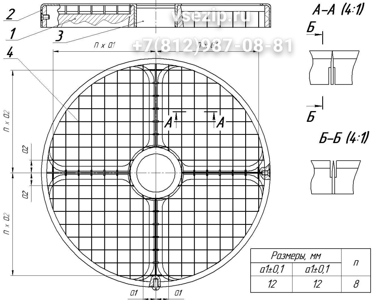
Рисунок 14 – Ножевая решетка
