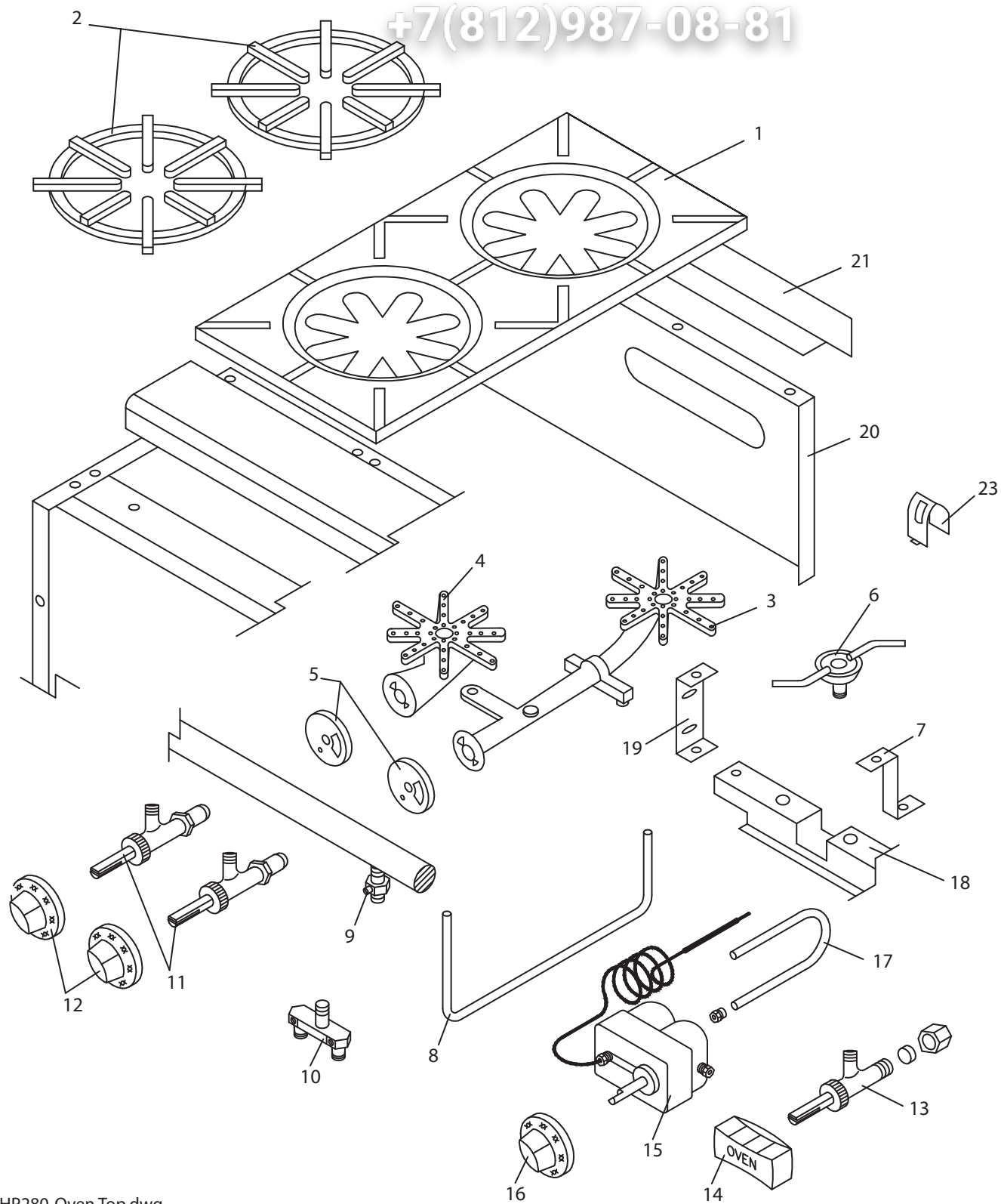
HP280-Oven Top.dwg
