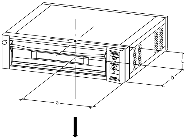
Fig. 5.2.Posizione del baricentro
