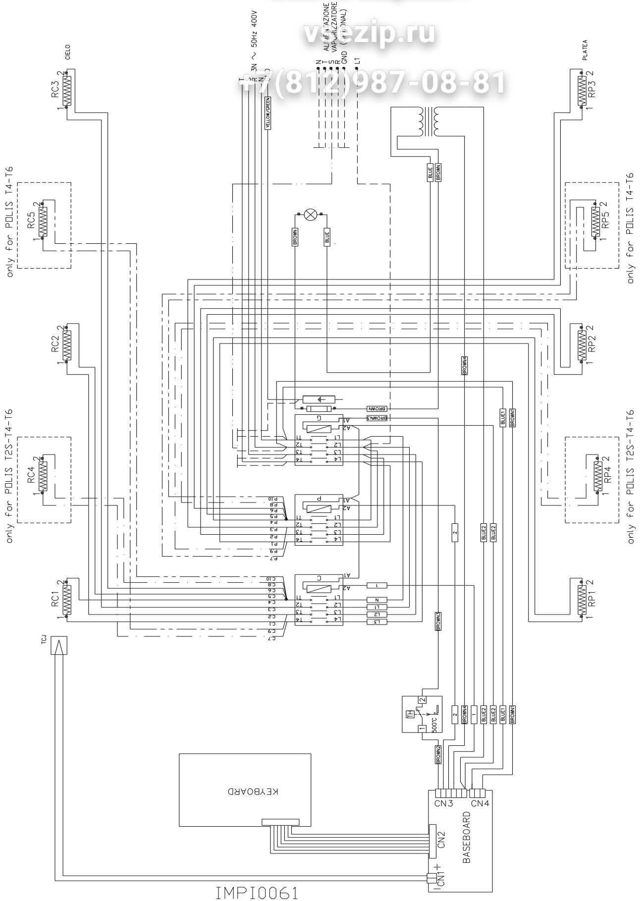
Fig.10-3 Schema elettrico a 400V 3-N
