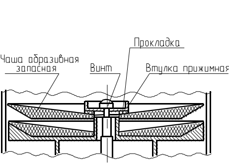
Рисунок 3 — Схема крепления чаши запасной абразивной
