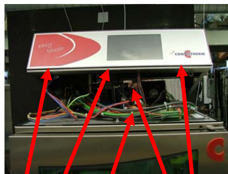
Панель управления easyToUCH ST7000 с сенсорным экраном (опция)
